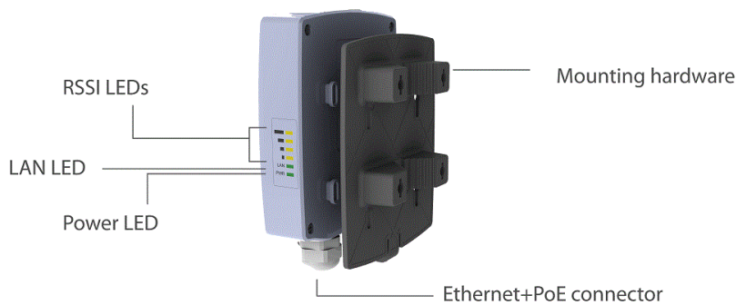
Figura 2 – Vista general del APC 5M-12 v2
