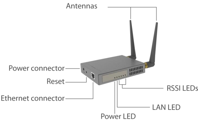
Figura 2 – Vista general del APC 2Mi
