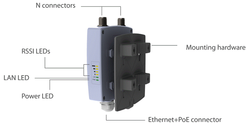
Figura 2 – Vista general del APC 2M
