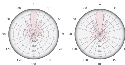
Patrón RF (vertical)
