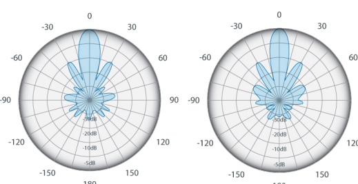
Patrón RF (horizontal)
